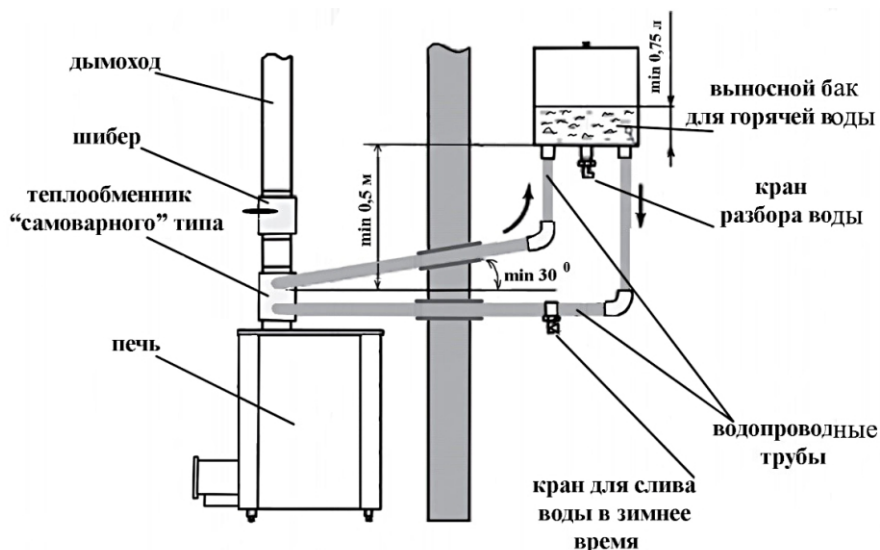
Рисунок 1 Схема монтажа теплообменника
