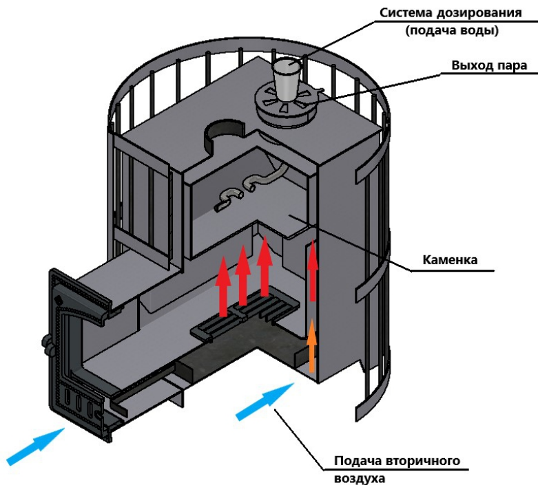
Рисунок 5 Банная печь EVEREST СПб™ из котловой стали 09Г2С схема работы печи
