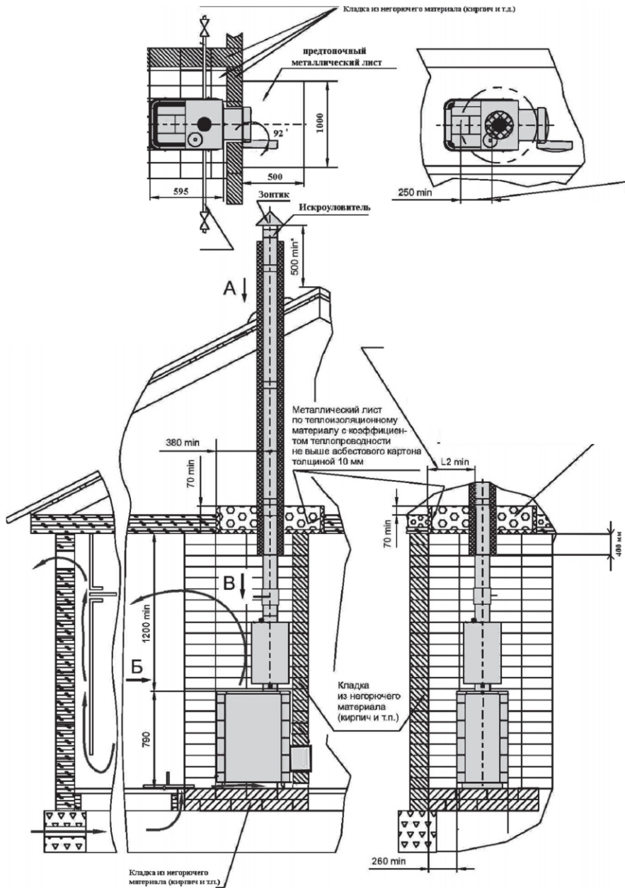
Рисунок 4 Схема монтажа печи
