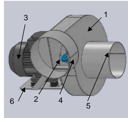
Рисунок 1 - Конструкция дымососа
