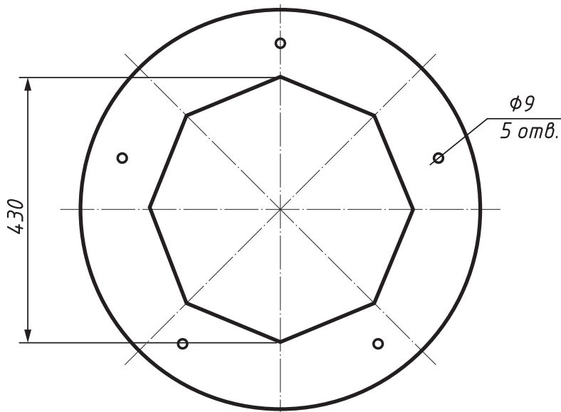
Рис. 2 Схема разметки на дне бочки отверстия под колосник и отверстий крепления зольного отсека.
